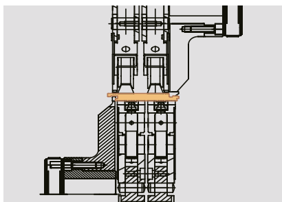
实木复合地板 — 窄链
