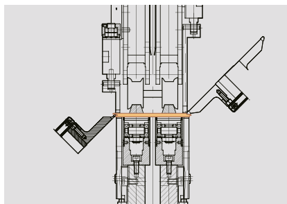
强化地板SPC — 双标准链
