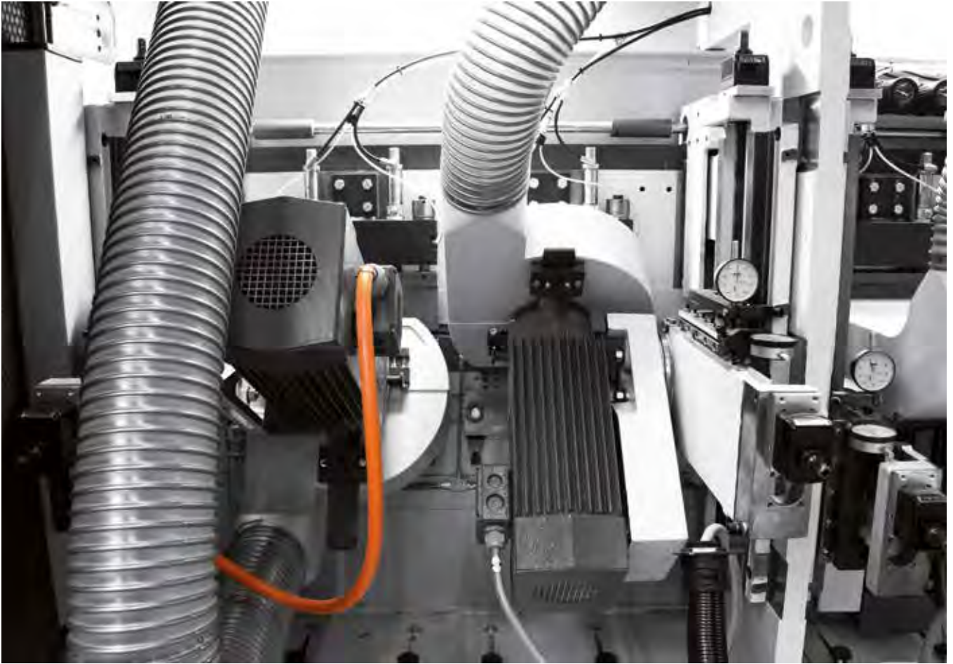
变频马达, 可以加工复杂的型材。
