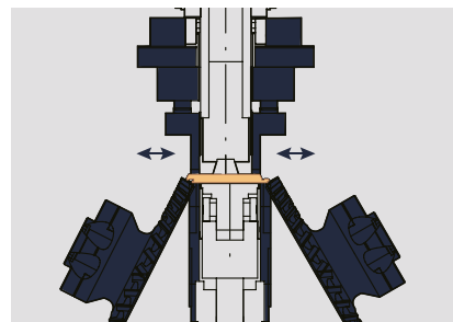
强化地板 — 单链
